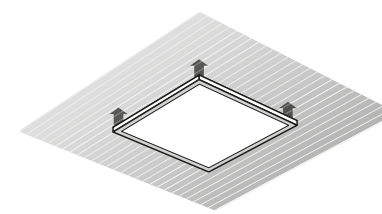
Рис. 2 Монтаж светильника накладным способом
