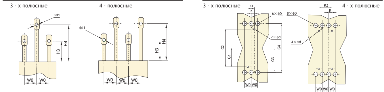
Разметка монтажной панели
