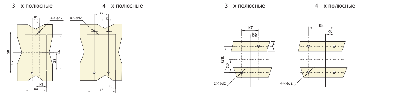
Разметка монтажной панели (M)
