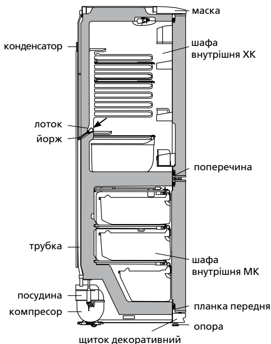
Рисунок 5 — Схема сливу талої води із ХК
