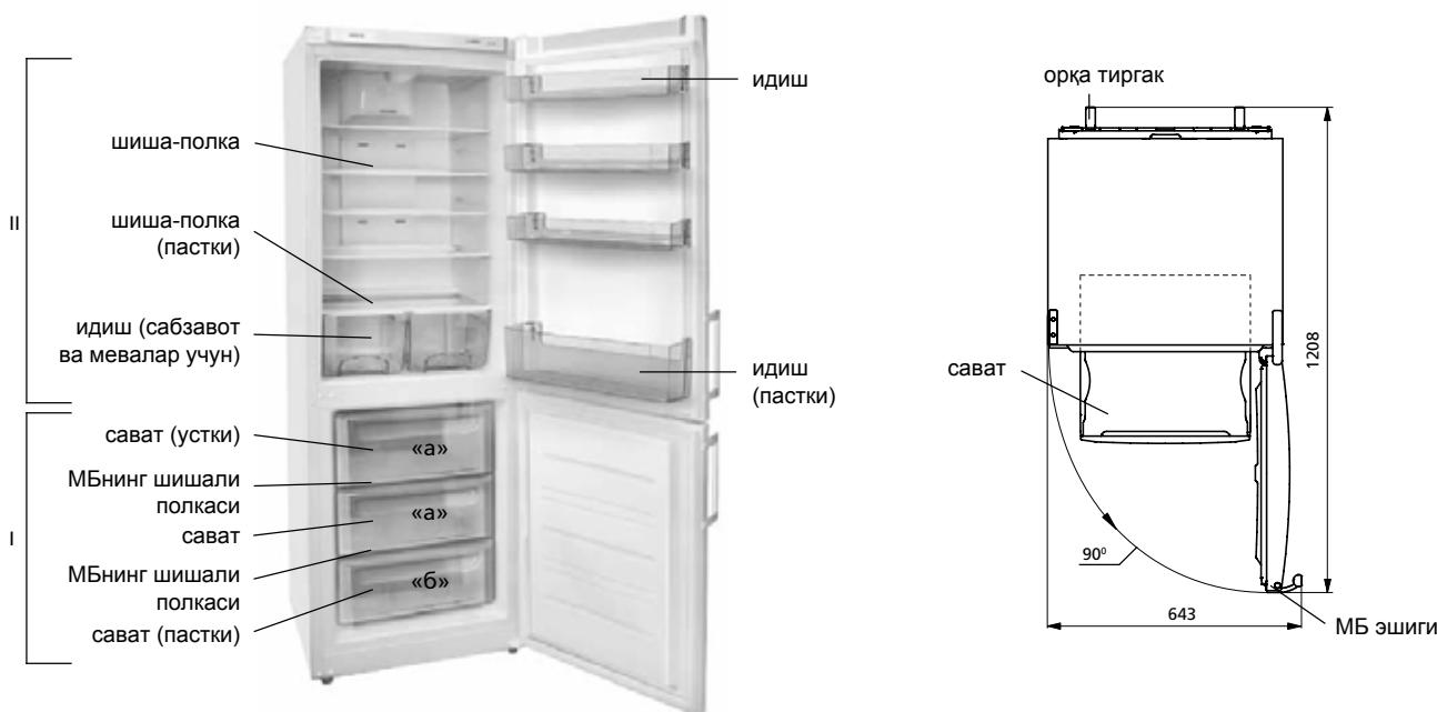
2-расм – Совутқич (уст қисмилан кўриниши)
