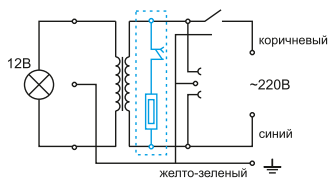
2. Светильник с подключением к сети 12 В
