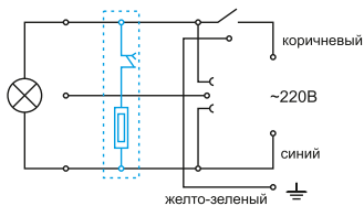
1. Светильник с подключением к сети ~220 В
