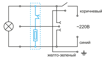
1. ~220 В желісіне жалғануы бар майшам
