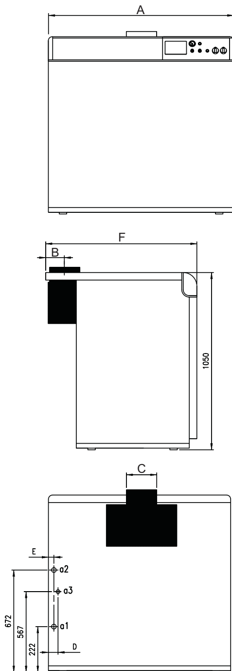
fig. 10 - Dimensions et raccords
