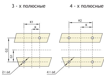
Разметка шин
