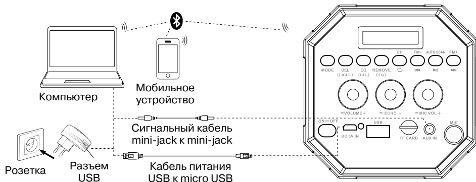
Рис. 2. Схема подключения
