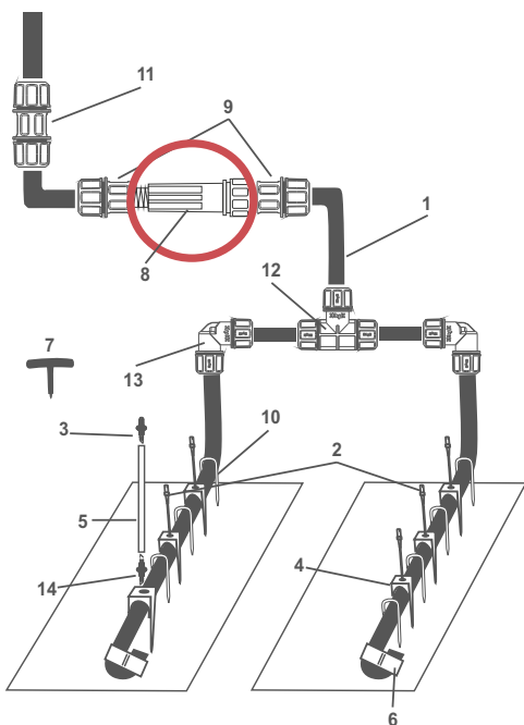
Рис. 1.1 Принципиальная схема сборки системы для 2-х грядок
