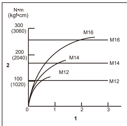
1. Време причвршћивања (секунде) 2. Момент причвршћивања
