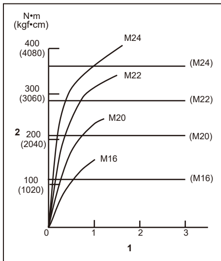
1. Vrijeme pričvršćivanja (u sekundama) 2. Zatezni moment
