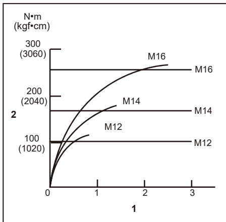
1. Време за стегање (секунди) 2. Вртежен момент
