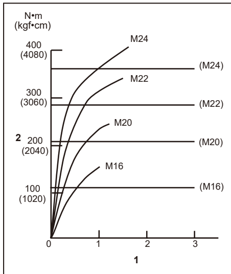
1. Час затягування (с) 2. Момент затягування
