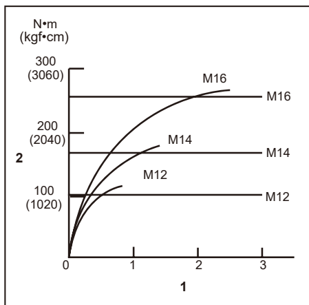
1. Čas privijanja (s) 2. Zatezni moment
