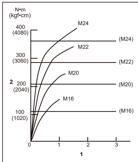
1. Време причвршћивања (секунде) 2. Момент причвршћивања
