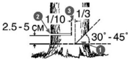
Рис. 11 Расположение запила, пропила и недопила
