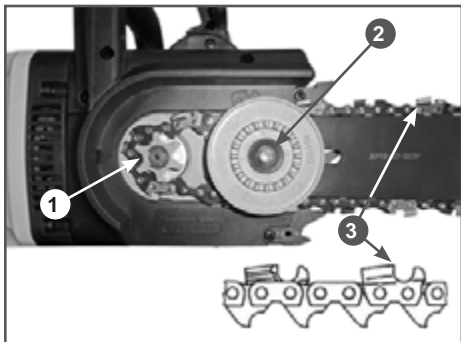
Рис. 5 Установка цепи
