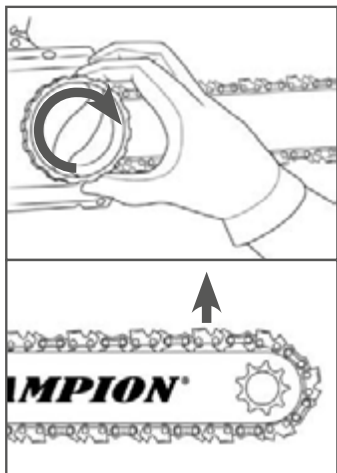
Рис. 7 Регулировка натяжения цепи
