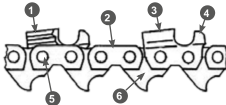
Рис. 17 Конструкция пильной цепи
