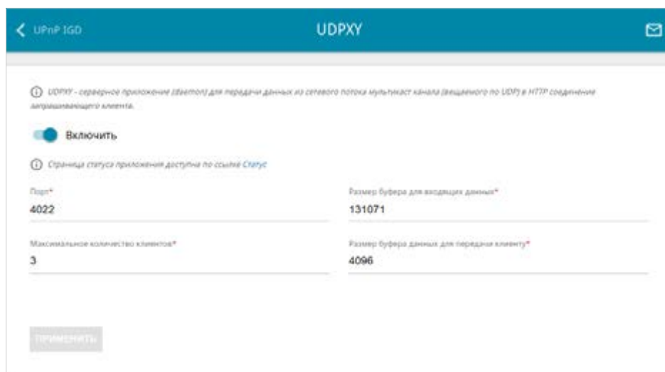
Рисунок 145. Страница Дополнительно / UDPXY .
