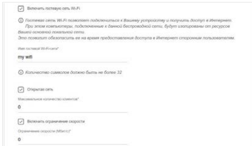
Рисунок 40. Страница настройки беспроводной сети.
