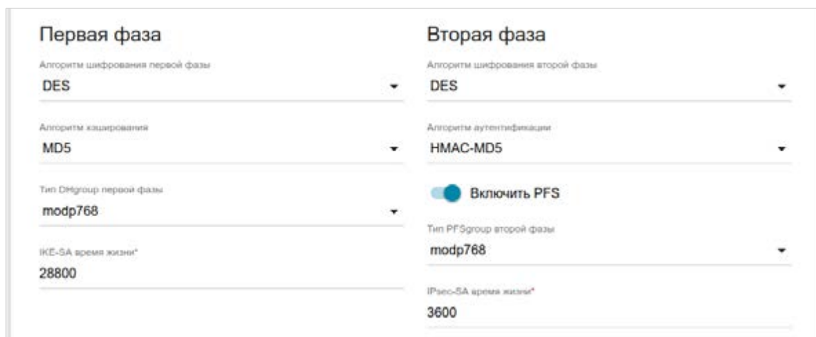
Рисунок 151. Страница добавления IPsec-туннеля. Разделы Первая фаза / Вторая фаза .
