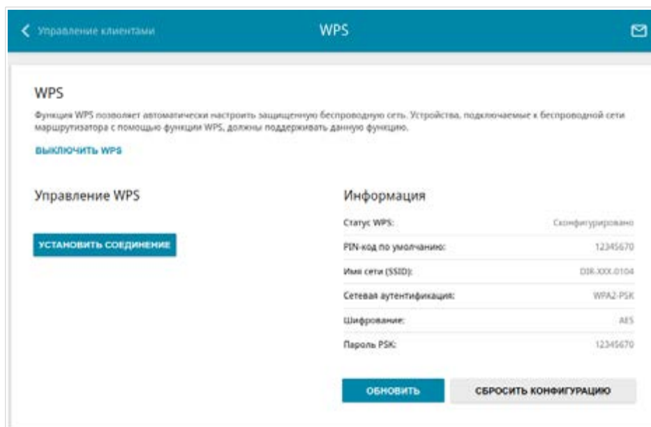
Рисунок 99. Страница для настройки функции WPS.
