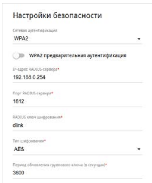
Рисунок 97. Значение WPA2 в раскрывающемся списке Сетевая аутентификация .
