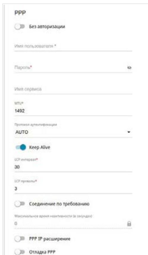
Рисунок 74. Страница добавления соединения типа PPPoE IPv6 . Раздел PPP .
