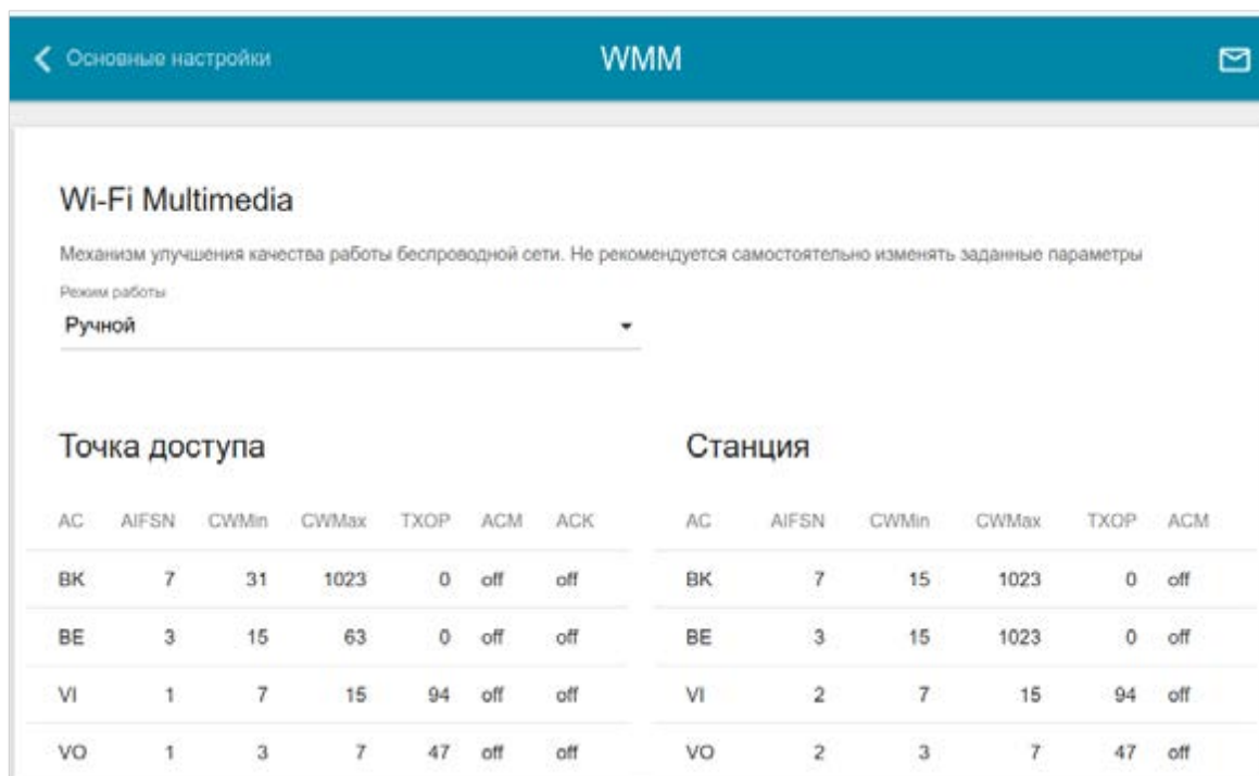
Рисунок 100. Страница для настройки функции WMM.
