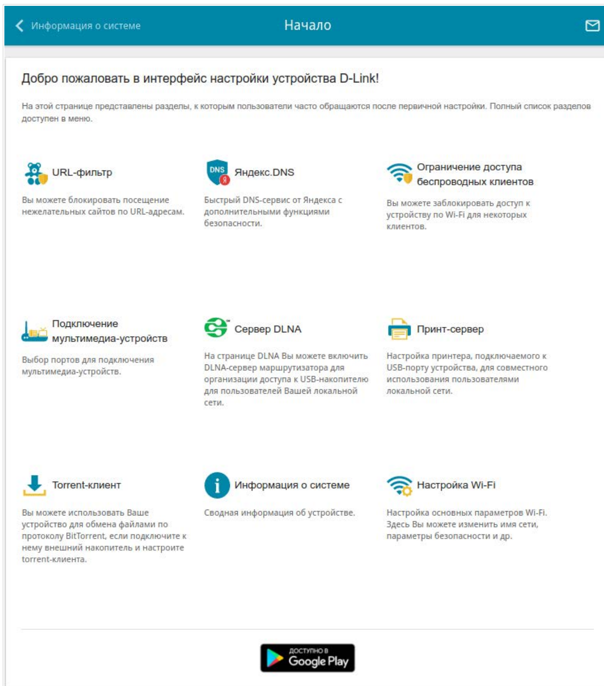
Рисунок 16. Страница Начало .
