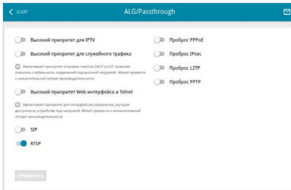
Рисунок 148. Страница Дополнительно / ALG/Passthrough .
