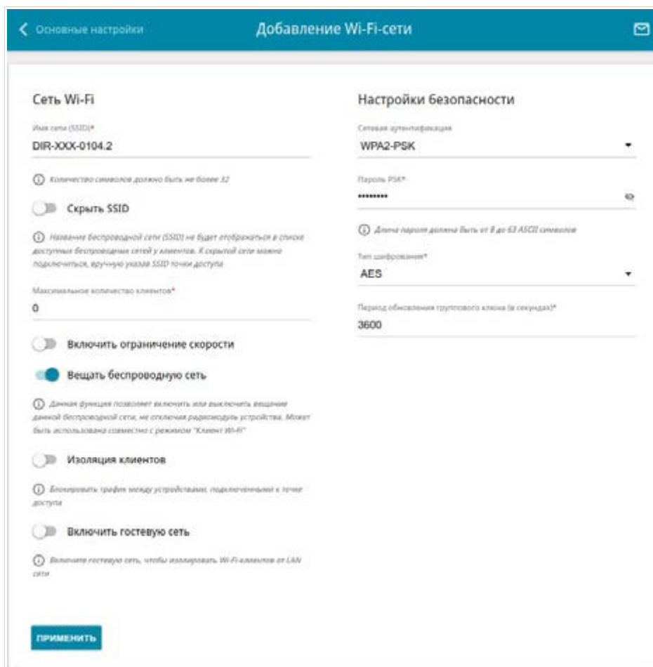
Рисунок 93. Создание беспроводной локальной сети.
