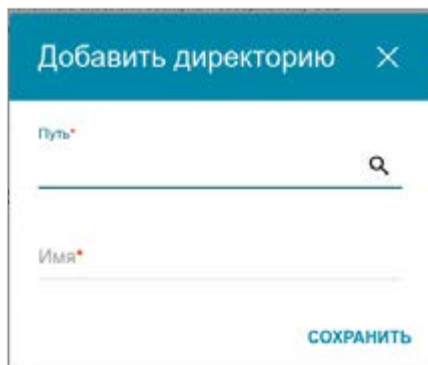
Рисунок 114. Добавление директории.
