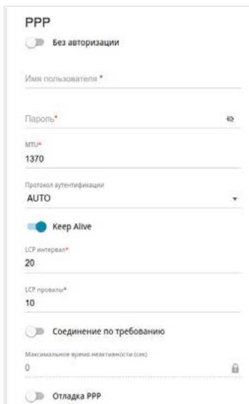
Рисунок 79. Страница добавления соединения типа 3G. Раздел PPP.
