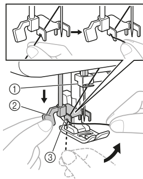
1 Иглодержатель 2 Рычажок нитевдевателя 3 Направляющая
