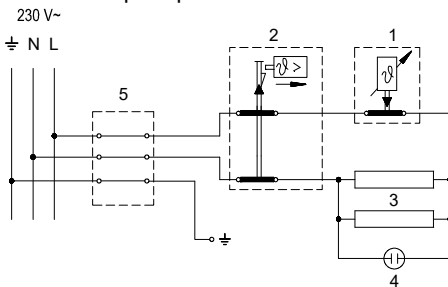
Электросхема
