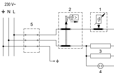
Instalația electrică
