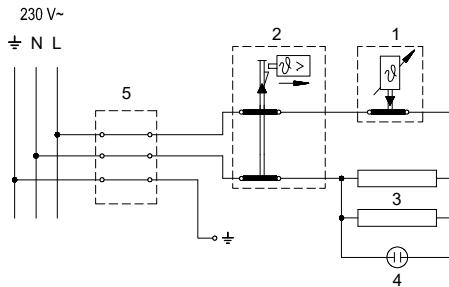
Електросхема
