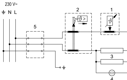
Šema povezivanja električnih provodnika
