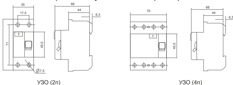
УЗО (2n)
