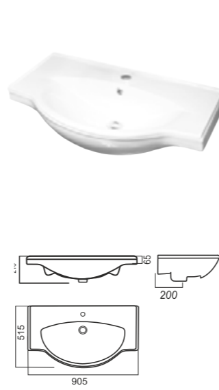
Умывальник CLASSIC 90
