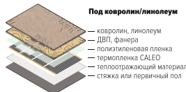
Рис. Схема монтажа теплого пола CALEO под ковролин или линолеум
