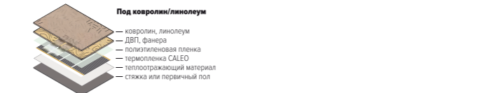
Рис. Схема монтажа теплого пола CALEO под ковролин или линолеум
