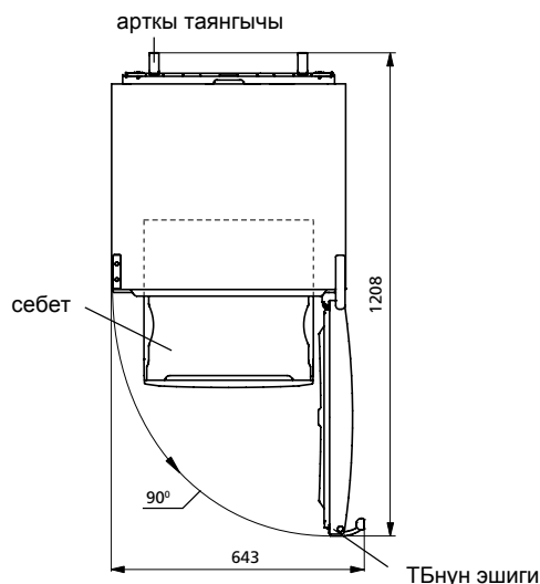
2-сүрөт – Муздаткыч (жогору жагынан көрүнгөн көрүнүшү)
