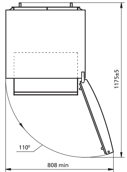
2-сүрөт – Муздаткыч (жогору жагынан көрүнгөн көрүнүшү)
