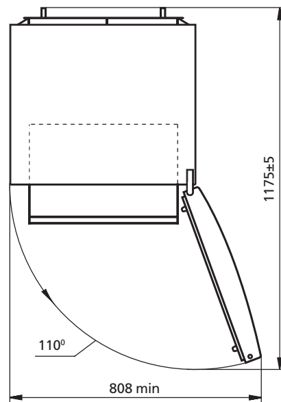
Рисунок 2 – Холодильник (вид сверху)
