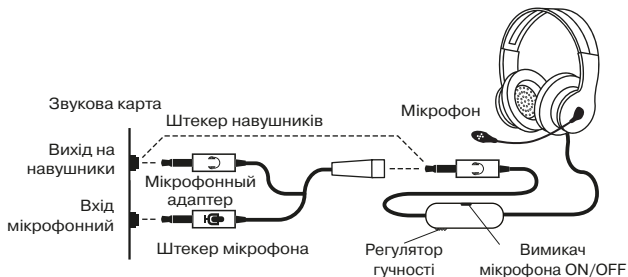
Мал. 1. Схема підключення
