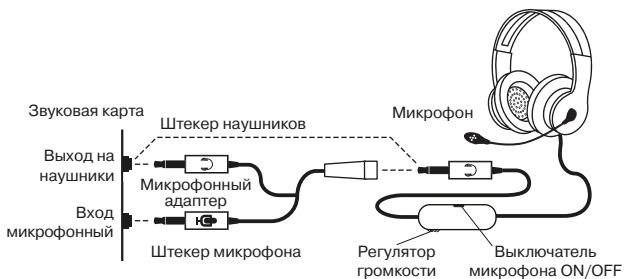
Рис. 1. Схема подключения
