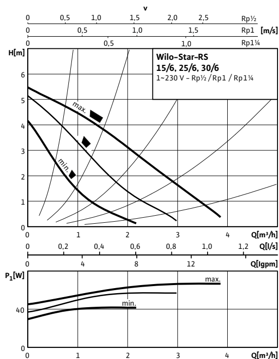
Wilo-Star-RS 15/6, 25/6, 30/6
